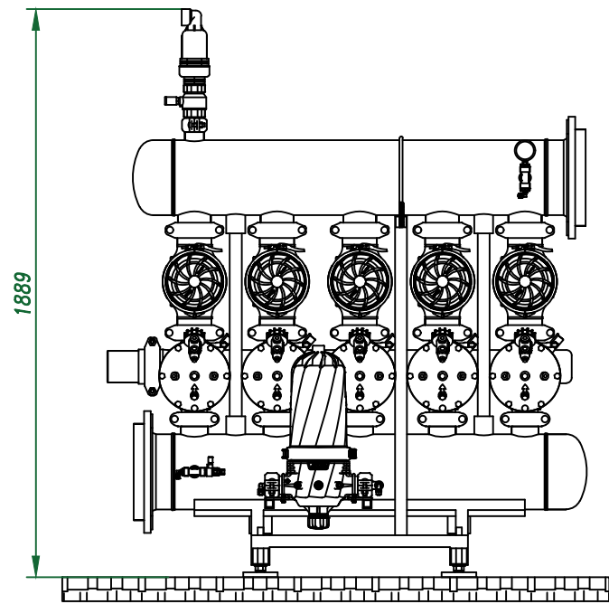
Вид спереди
